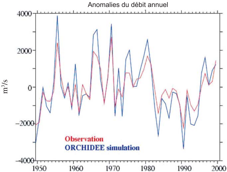
Figure 4.13 Comparaison entre observation et simulation pour le débit du Danube au cours de la période historique.
