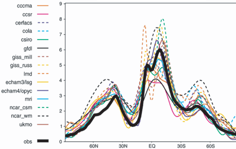
Figure 4.8 Répartition zonale des précipitations moyennes (en mm/jour) d'hiver (décembre à février), pour le climat actuel, telles que simulées par les modèles engagés dans l'expérience d'intercomparaison CMIP1. Les valeurs mesurées sont représentées par la courbe en trait fort (d'après Lambert et Boer, 2001).
