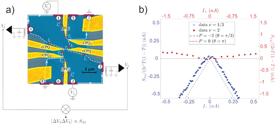
Figure 9. a) Image au microscope électronique de l'échantillon collisionneur d'anyons. Un courant électrique continu est généré aux contacts 1 et 2. Deux CPQ (CPQ1 et CPQ2) sont utilisés comme émetteurs aléatoires d'anyons qui se propagent vers le troisième CPQ (cCPQ) utilisé comme lame séparatrice dans la collision. On mesure les corrélations croisées des fluctuations des courants électriques en sortie de la lame séparatrice en fonction du courant total d'anyons généré, I_+ = I_1 + I_2 . b) Corrélations croisées S_{34} normalisées par le facteur 2e^*T(1 - T) (avec e^* = e/3 dans le régime fractionnaire et e^* = e dans le régime entier) en fonction du courant I_+ . Dans le régime entier, on observe des corrélations légèrement positives et proches de 0, P \approx 0 , caractéristiques de l'exclusion des fermions. Dans le régime fractionnaire, on observe des corrélations très négatives ( P \approx -2 ) qui traduisent le regroupement d'anyons formant des paquets de charge dans une sortie de la lame séparatrice.
